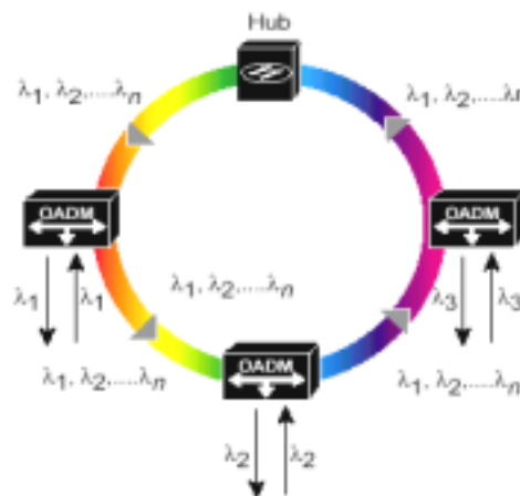
Fig. 15 – Topologia em anel
