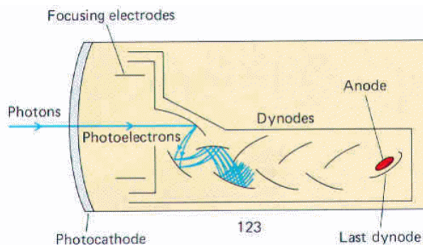
Figura 6.17: Esquema de funcionamento de uma fotomultiplicadora.
