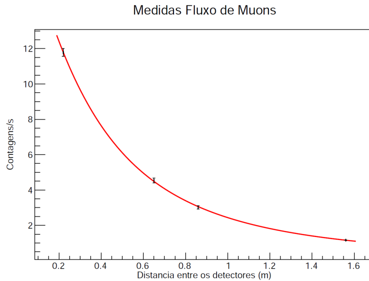
Figura 6.37: Dependência da frequência de contagens com a distância entre os detectores.
