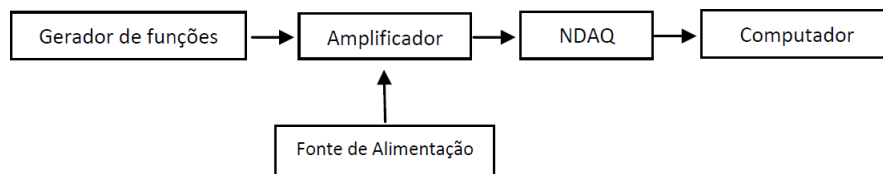
Figura 6.12: Esquema experimental para calibração do amplificador.
