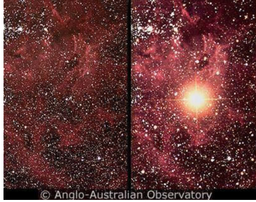
Figura 2.11: Supernova SN1987A, céu antes e após a Supernova respectivamente.
