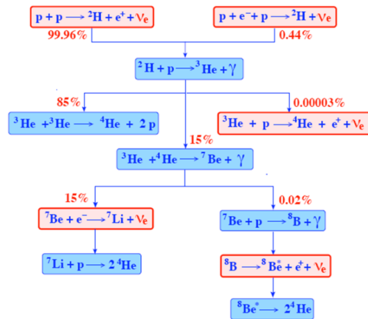
Figura 2.2: Cadeia de reações pp.
