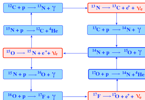
Figura 2.3: Ciclo CNO.
