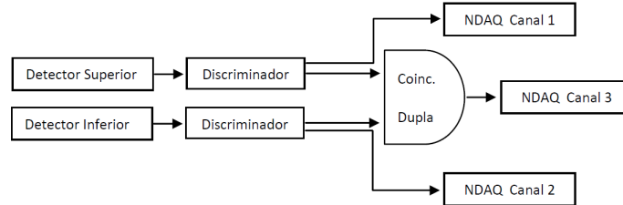
Figura 6.33: Esquema experimental para aquisição das coincidências duplas no detector cintilador.
