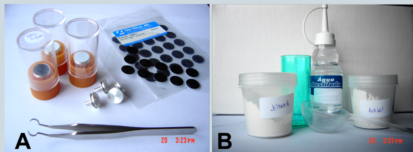
(A) Método tradicional de “stub” e fita condutora dupla face e (B) material para luva de resina poliéster
