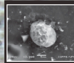
Fig. 2: Partícula resultante da deflagração da oer 8mm e espectro de EDS
