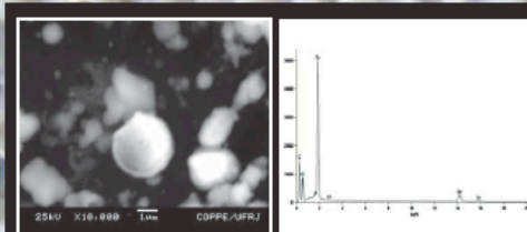
Fig. 1: Resíduos de tiro de munição CBC CleanRange e respectivo espectro EDS
